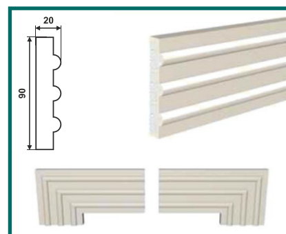
МД-90/1 (90 × 20 × 2000)
