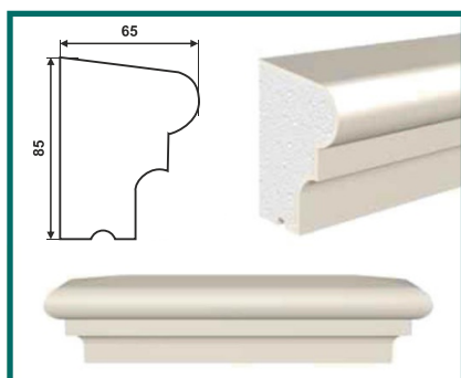
ПК-85/1 (85 × 65 × 2000)
