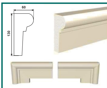
МД-130/2 (130 × 60 × 2000)
