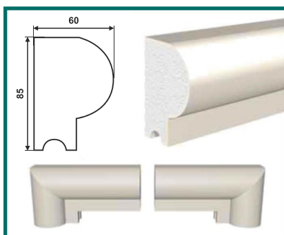
МД-85/2 (85 × 60 × 2000)
