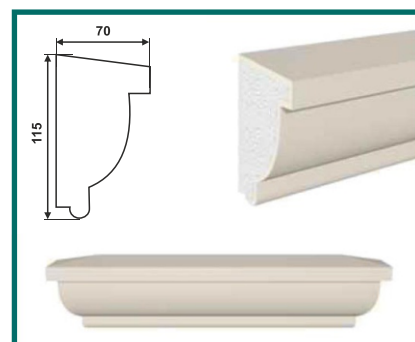
ПК-115/1 (115 × 70 × 2000)
