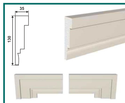
МД-130/3 (130 × 35 × 2000)
