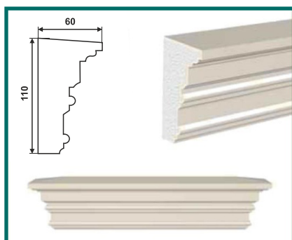
ПК-110/2 (110 × 60 × 2000)
