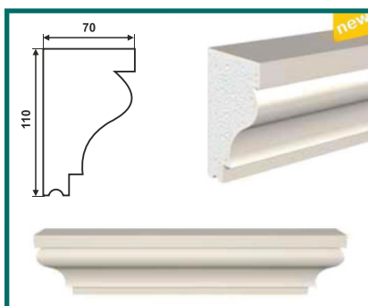
ПК-110/3 (110 × 70 × 2000)
