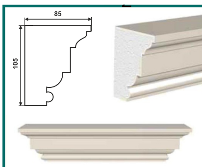
ПК-105/1 (105 × 85 × 2000)
