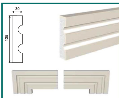
МД-135/1 (135 × 30 × 2000)
