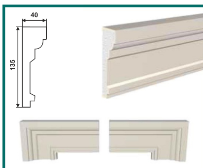
МД-135/2 (135 × 40 × 2000)
