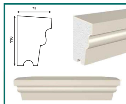
ПК-110/1 (110 × 75 × 2000)
