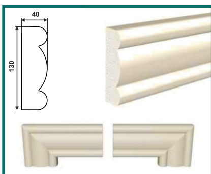
МД-130/1 (130 × 40 × 2000)
